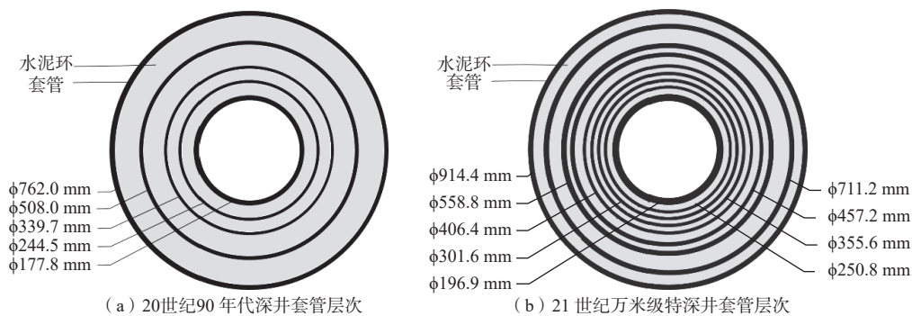
图 3 墨西哥湾深井及万米级特深井的套管层次
