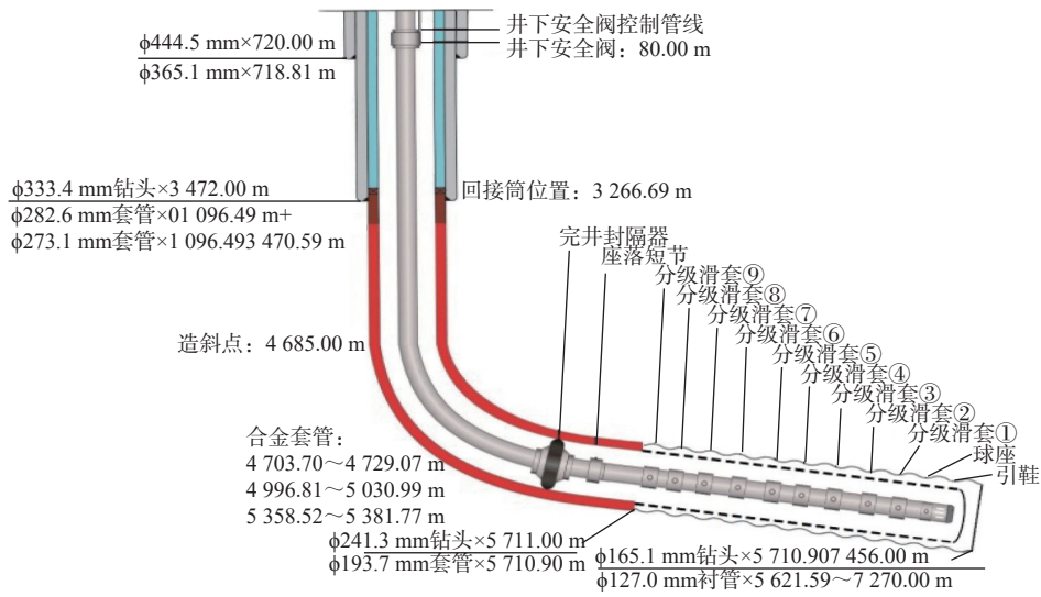
图 4 超深长水平段水平井滑套分流完井试气管柱
