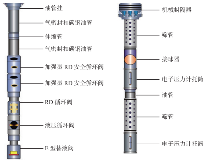
图 1 超深层油气井加强型“五阀一封”测试管柱示意
