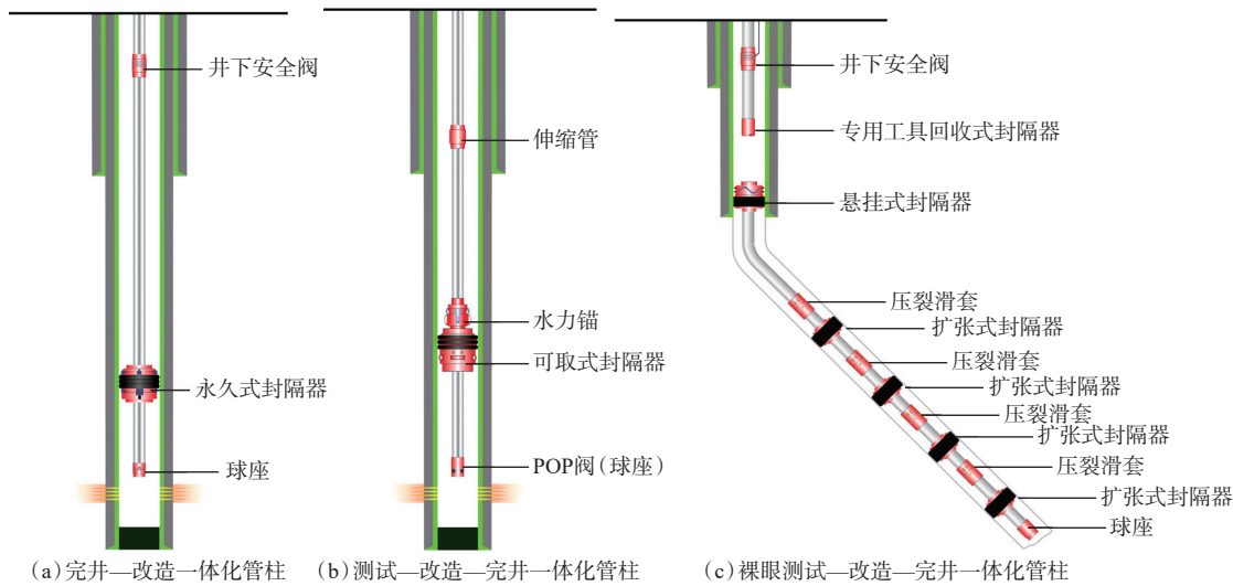
图 2 超深层油气井测试—改造—完井一体化管柱示意
