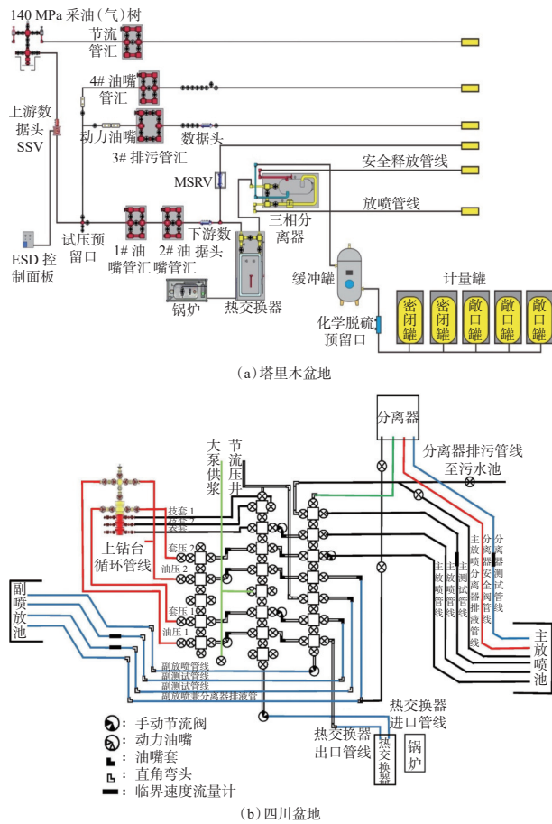
图 6 中国石化“深地工程”地面测试流程示意
