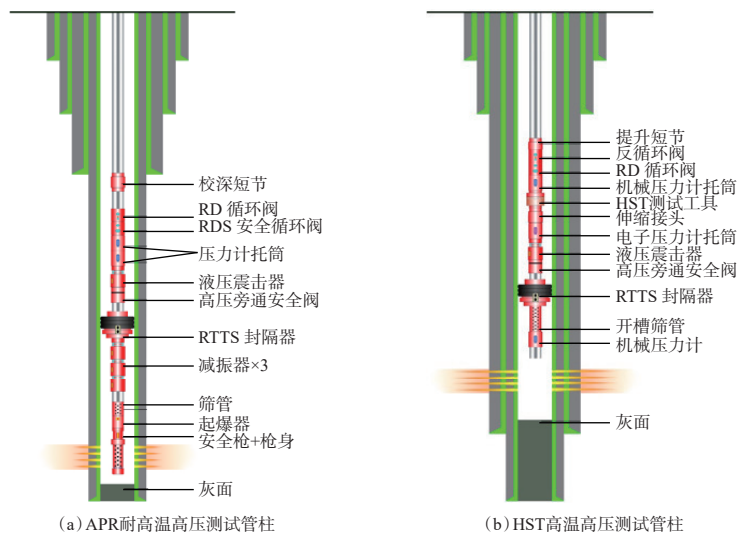
图 5 准噶尔盆地深层砾岩储层油气测试技术管柱
