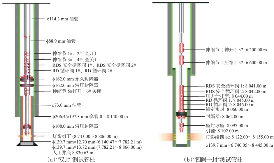
图3 超深高酸性油气藏联作测试管柱
