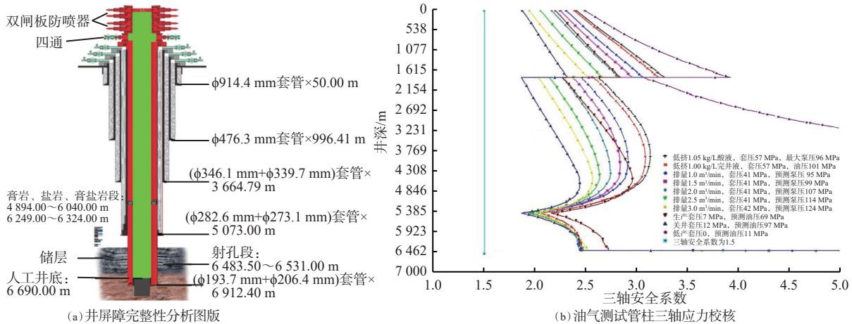
图 7 窄安全窗口油气井测试工程设计技术
