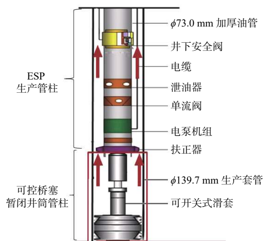
图3 可控桥塞完井管柱示意
