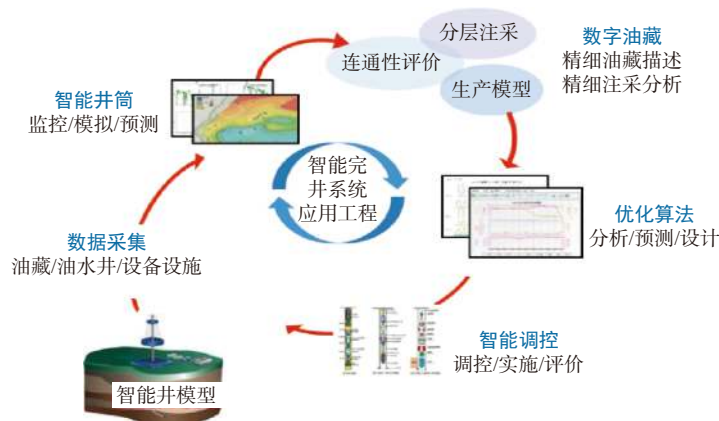
图 6 油藏生产动态优化和精细化管理系统基本原理
