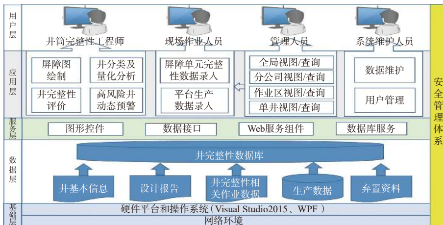
图 3 海上油气井完整性管理系统架构
