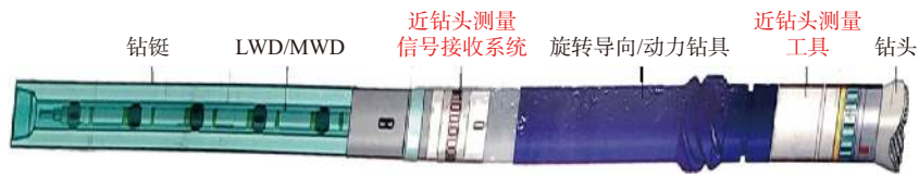
图 2 井下钻井参数测量及信号短传系统在钻具组合中的位置
