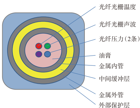
图 4 光纤光缆横截面结构
