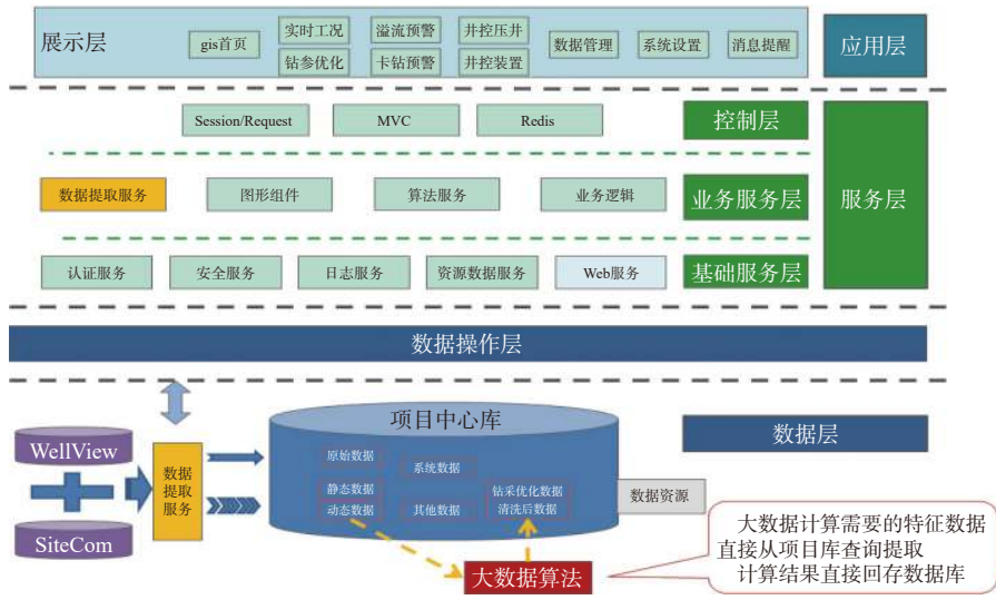
图 1 深水钻井大数据在线分析软件架构
